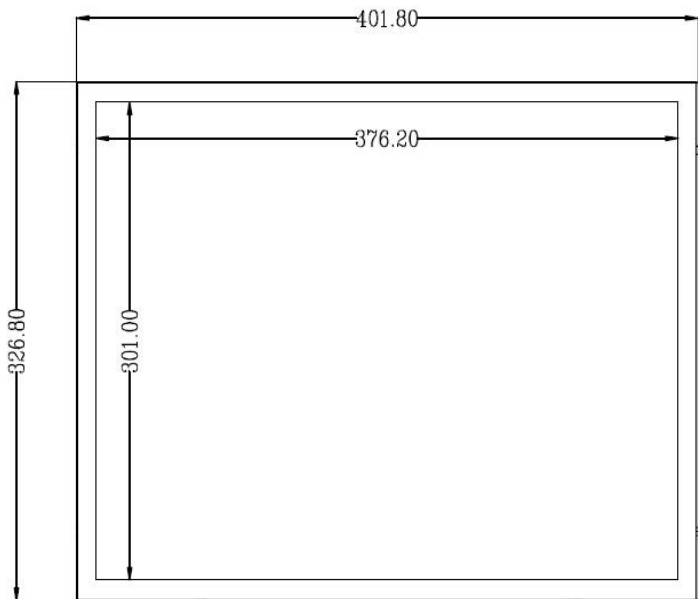
19寸 (MT190EN02) 监视器外形
